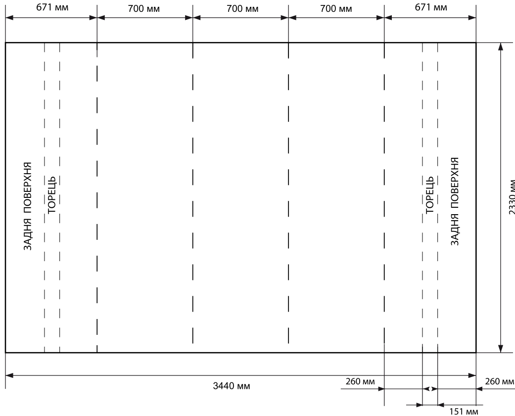
ВИД СВЕРХУ
